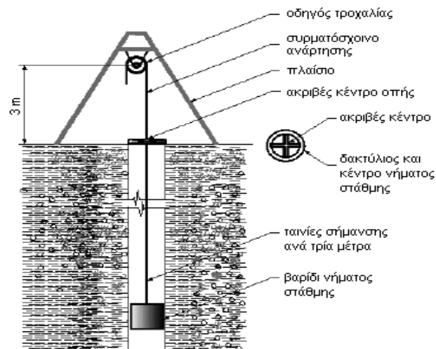
Σχήμα 2 - Διάταξη ελέγχου κατακορύφωσης υδρογέωτρησης
