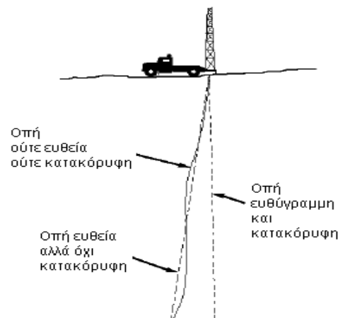
Σχήμα 1 - Τύποι αποκλίσεων υδρογέωτρησης
