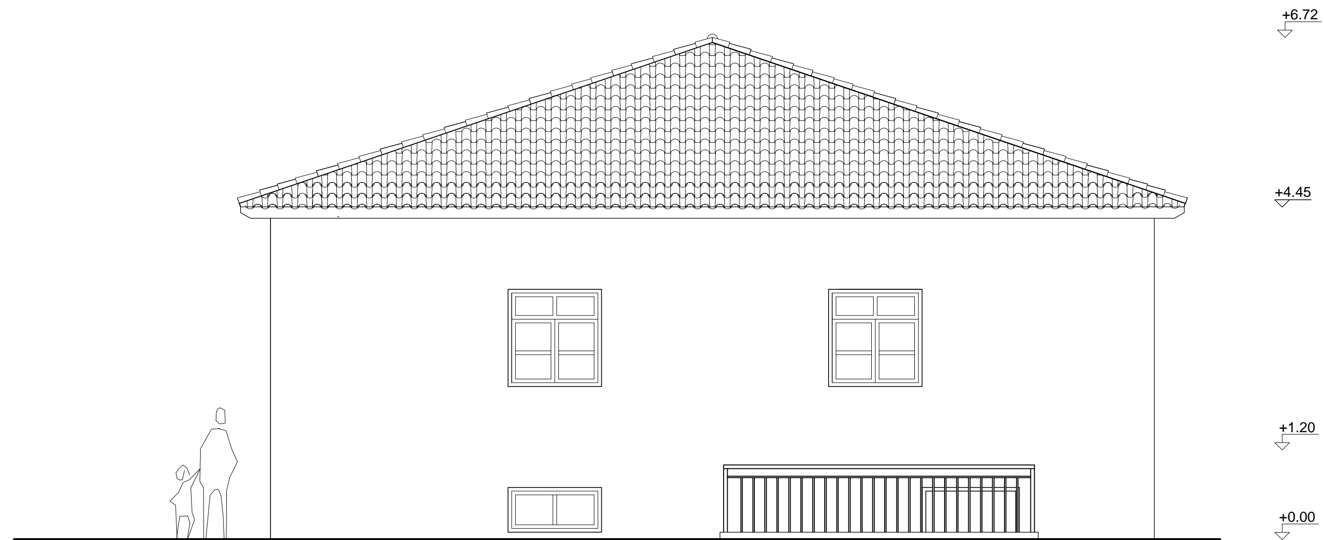
ΝΟΤΙΟΑΝΑΤΟΛΙΚΗ ΟΨΗ
